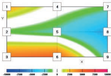
Rastermessung magnetischer Gleichfelder in nT
